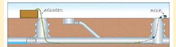
マンホールから既存の管に新管材をいれる。
